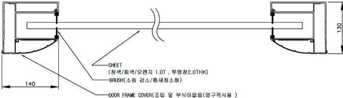
<KAD-2500 가이드레일 단면도>
