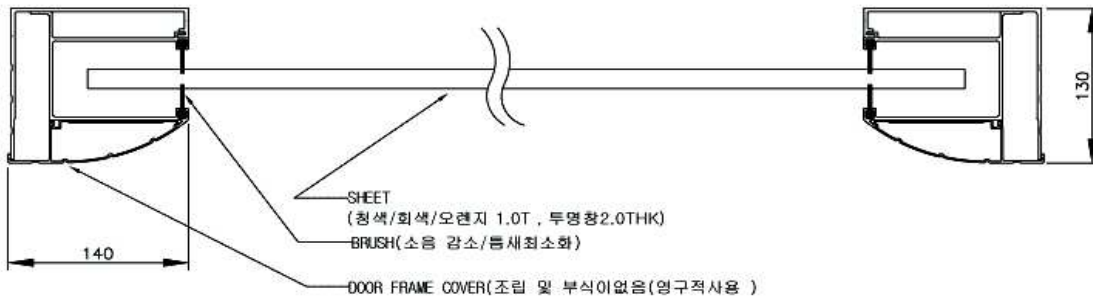
<KAD-2500 가이드레일 단면도>
