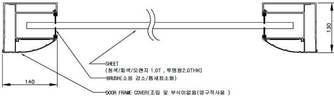
<KAD-2000 가이드레일 단면도>
